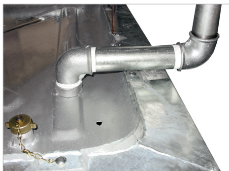
Belüftungsanschluss
